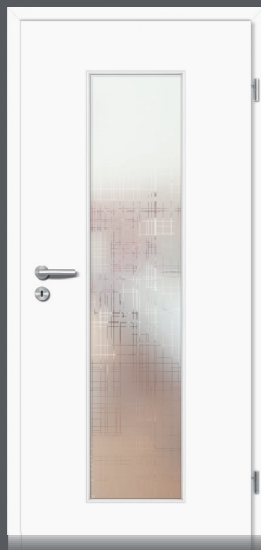
Holztür mit Lichtausschnitt LA3 verglast mit PANNO CPL Weißlack 9016 Maße 860/1985/145 mm Gefälzte Tür, Rundkantenzarge FU-RF Mögliche Beschläge SOFT, RAVENNA o. QUADRAL in Edelstahl matt
